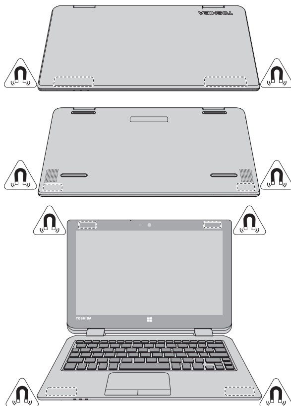
Obrázek 3-14 Umístění magnetů (CL10W-B/L10W-B)
