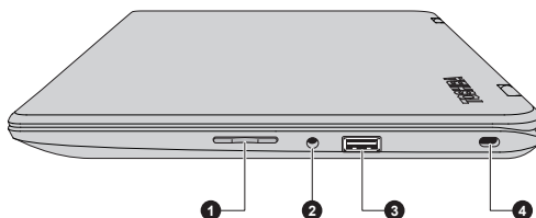
Obrázek 3-10 Pravá strana počítače (CL10W-B/L10W-B)
