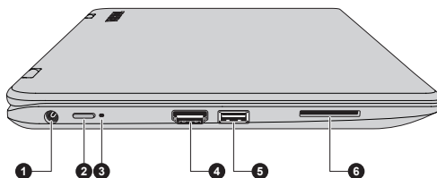
Obrázek 3-9 Levá strana počítače (CL10W-B/L10W-B)
