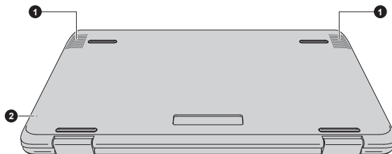
Obrázek 3-12 Spodní strana počítače (CL10W-B/L10W-B)
