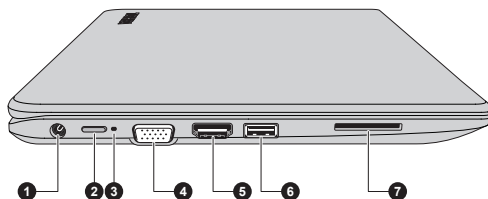
Obrázek 3-2 Levá strana počítače (CL10-B/L10-B)
